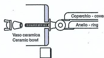
Cerniere per vaso con fori orizzontali Hinges for vase with horizontal holes
